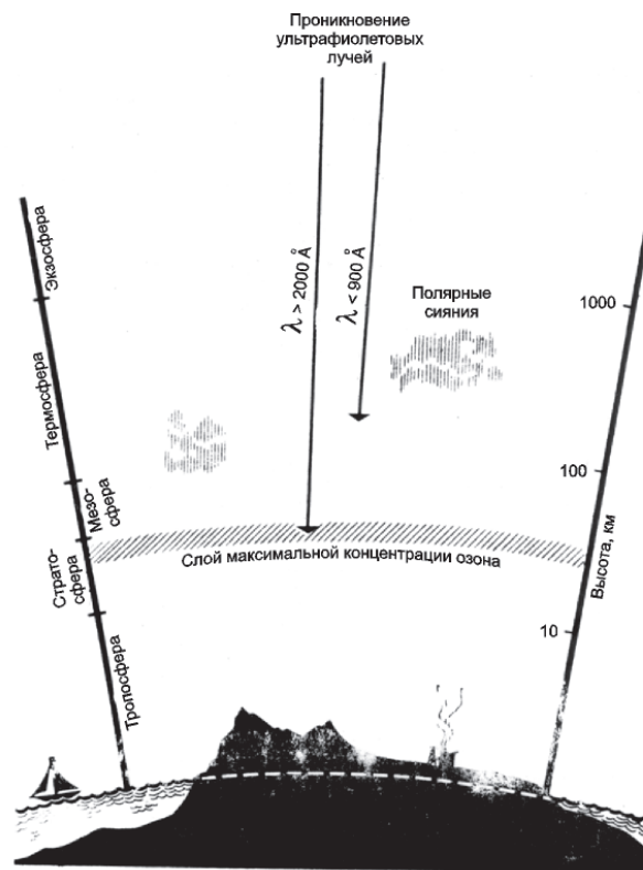
Рисунок 15.27 — Озоновый слой Земли
