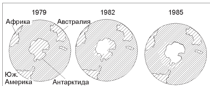
Рисунок 16.4 — Озоновая дыра (по Н. Ф. Реймерсу, 1990)
