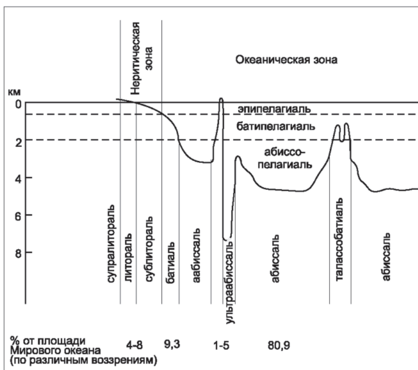
Рисунок 5.2 — Вертикальная экологическая зональность океана (по Н. Ф. Реймерсу, 1990)
