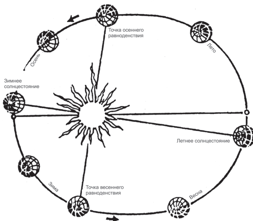
Рисунок 10.1— Путь Земли вокруг Солнца
